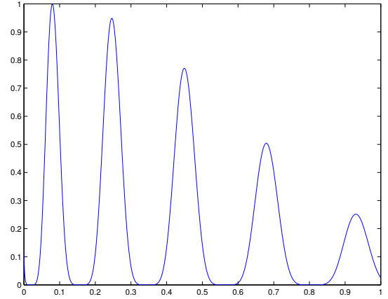
Fig. 3. Uneven Decreasing Maxima.
