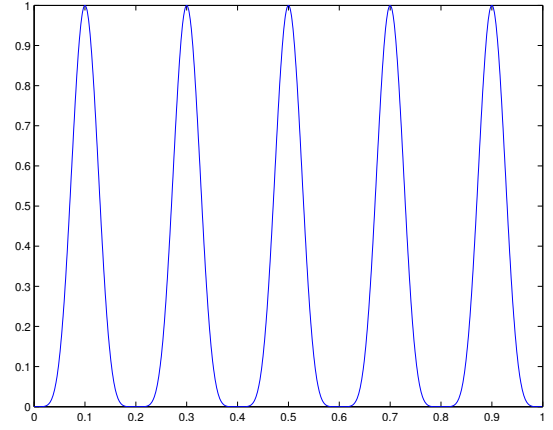
Fig. 2. Equal Maxima.
